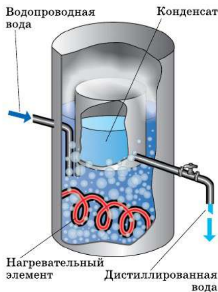
Рис. 63. Устройство дистиллятора
