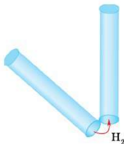
Рис. 44. «Переливание» водорода
