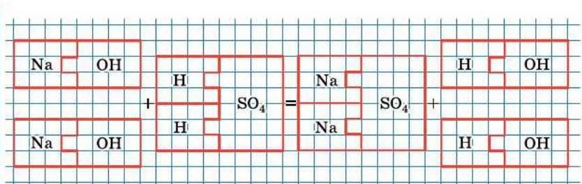
Рис. 79. Составление уравнения реакции нейтрализации из бумажных моделей
