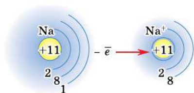
Рис. 90. Атом натрия и катион натрия. Радиус иона меньше радиуса атома, так как ион содержит меньше занятых энергетических уровней
