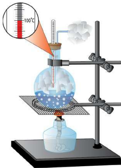
Рис. 7. Определение температуры кипения жидкости
