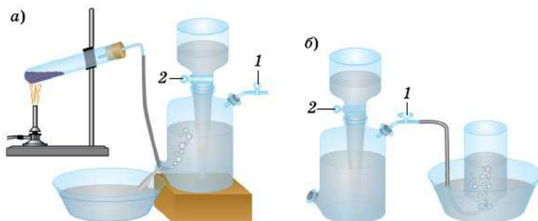
Рис. 32. Газометр: а — заполнение газометра кислородом (краны 1, 2 закрыты); б — наполнение сосуда кислородом из газометра (краны 1, 2 открыты)
