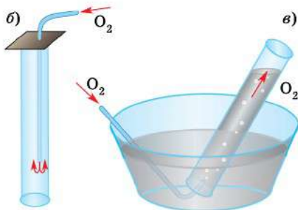
Рис. 31. Получение кислорода разложением пероксида водорода (а) и его собирание вытеснением воздуха (б) и над водой (в)
