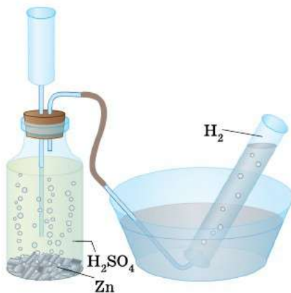
Рис. 46. Прибор для получения водорода
