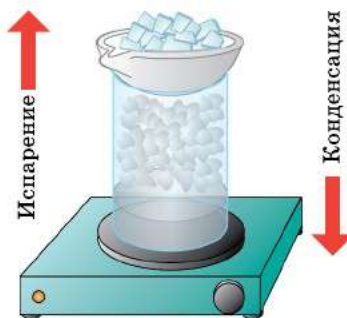
Рис. 12. Испарение и конденсация этилового спирта
