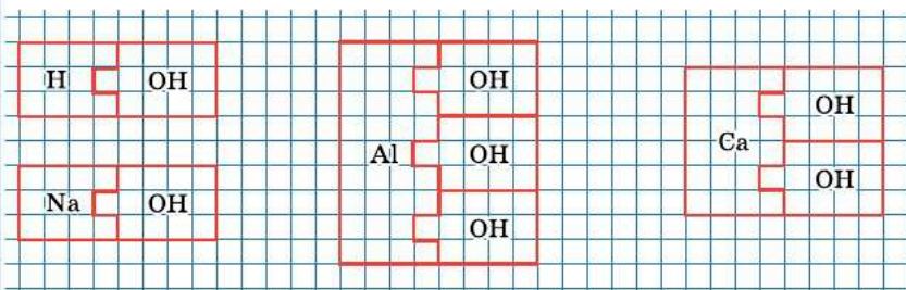
Рис. 75. Составление бумажных моделей воды и оснований
