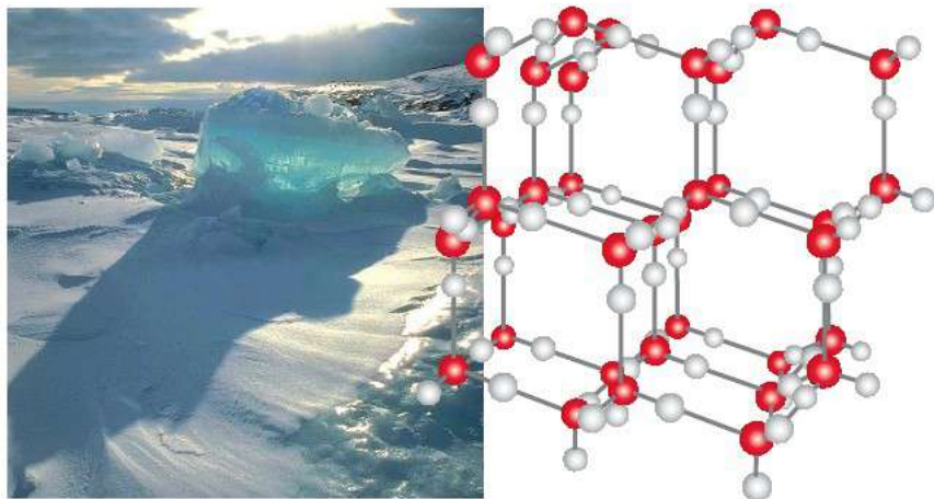
Рис. 116. Фрагмент кристаллической структуры льда. Между молекулами воды существуют слабые водородные связи
