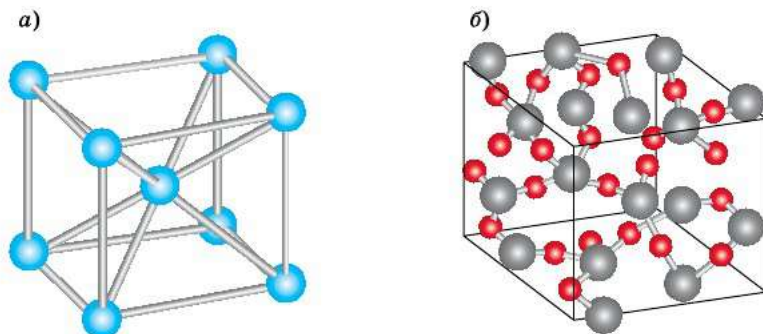
Рис. 23. Строение некоторых веществ: а — железа; б — кварца
