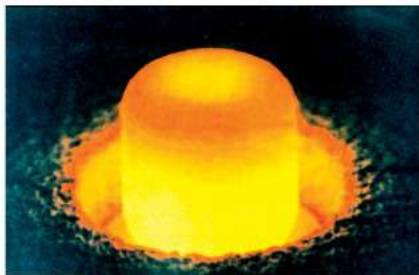
Рис. 86. Радиоактивный металл кюри светится в темноте, испуская большое количество ядер гелия
