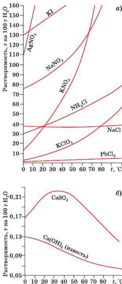
Рис. 66. Кривые растворимости некоторых веществ
