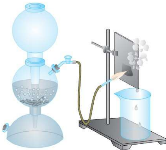
Рис. 50. Горение водорода на воздухе
