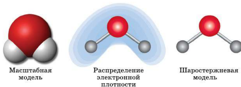
Рис. 99. Различные модели молекулы воды
