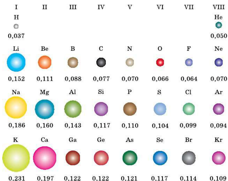
Рис. 92. Радиусы атомов некоторых химических элементов в нанометрах, нм ( 1 \text{ нм} = 10^{-9} \text{ м} )
