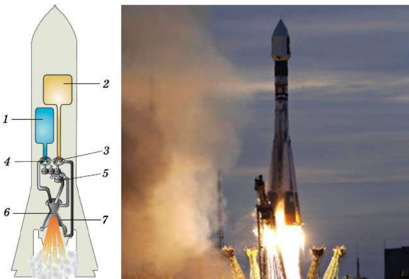
Рис. 41. Ракетный двигатель. Окислитель — жидкий кислород 1 и горючее — керосин или жидкий водород 2 из баков-хранилищ насосами 3, 4 при помощи турбины 5 подаются в камеру сгорания 6. Наружная её часть представляет собой реактивное сверхзвуковое сопло 7, в котором газы, образовавшиеся при сгорании топлива, разгоняются до скорости, превышающей скорость звука. Ракета движется за счёт выброса газов
